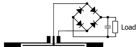
(d) Circuit used in experiments (b) and (c).
